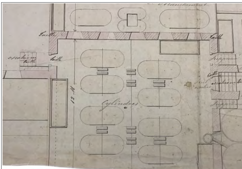
77 J 155, Fonds papeteries Vallée, plan technique de l'usine (détail), 1882 : la salle des cylindres.
