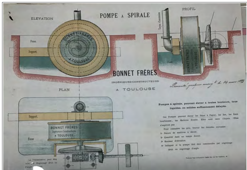
77 J 159, Fonds papeteries Vallée, plans techniques de pompe à spirale, document promotionnel, 1883.
