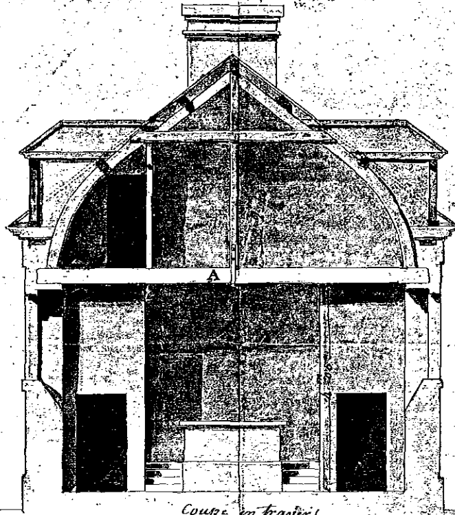
Coupe en travers.
